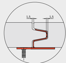
Rozmiar szczeliny przy maksymalnym wydłużeniu
