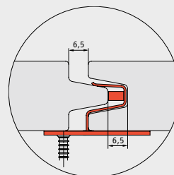
Rozmiar szczeliny przy montażu za pomocą klamer montażowych
